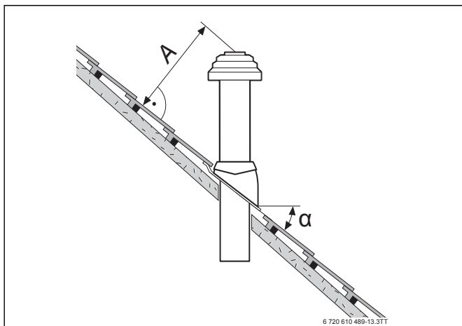
Рис. 6 Расстояния и углы наклона крыши
