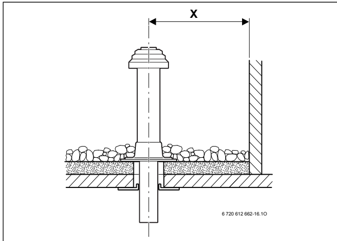
Рис. 5 Расстояния для плоской крыши
