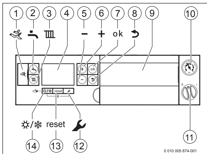
Рис. 32 Панель управления с открытой крышкой
