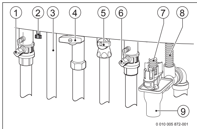
Рис. 27 Подключения газа и воды (дополнительная комплектация)
