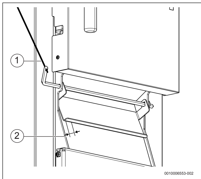
Рис. 3 Регулировка натяжения цепи
