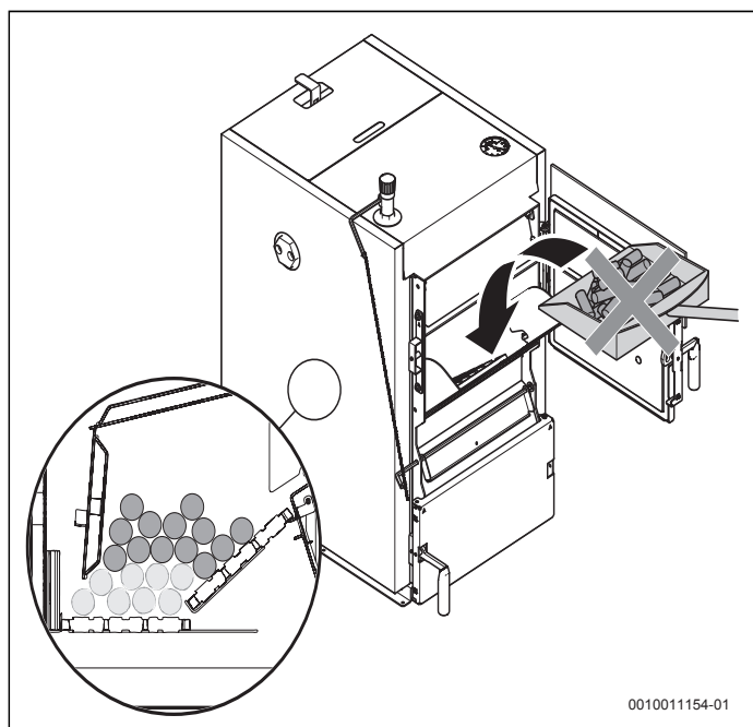
Рис. 11 Загрузка небольшого количества топлива
