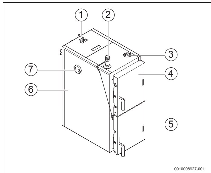
Рис. 1 Функциональные элементы котла
