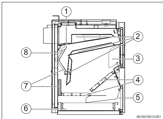
Рис. 2 Внутреннее устройство котла (показан в разрезе)
