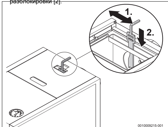
Рис. 6 Закрытие растопочной заслонки
