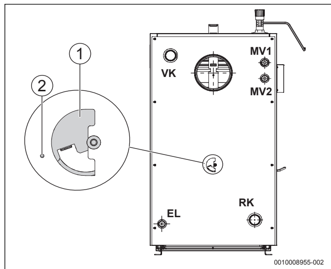
Рис. 4 Регулировка заслонки вторичного воздуха [1] Заслонка вторичного воздуха [2] Метка
