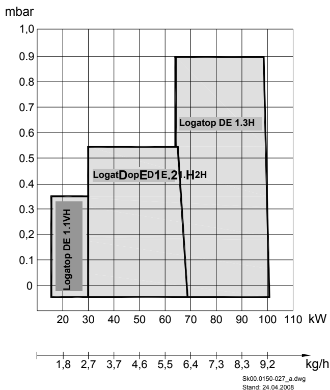
Рис. 15: Рабочий диапазон Logatop DE1.. Описание:
