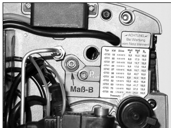
Рис. 8: Установка значений V и ниппель измерения напора воздуха создаваемого вентилятором
