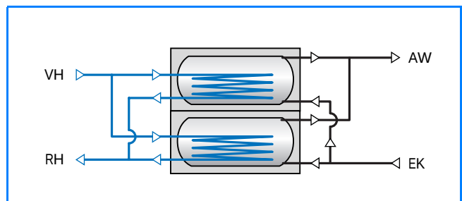
7/1 Принцип работы двух параллельно подключенных емкостных водонагревателей (гидравлические соединения выполнены по „системе Тихельмана“)
