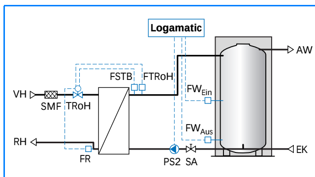
15/1 Принцип регулирования для системы с промежуточным теплообменником с одним загрузочным насосом и двумя датчиками температуры при непосредственном нагреве от теплоцентрали (питание через регулятор температуры без вспомогательной энергии)
