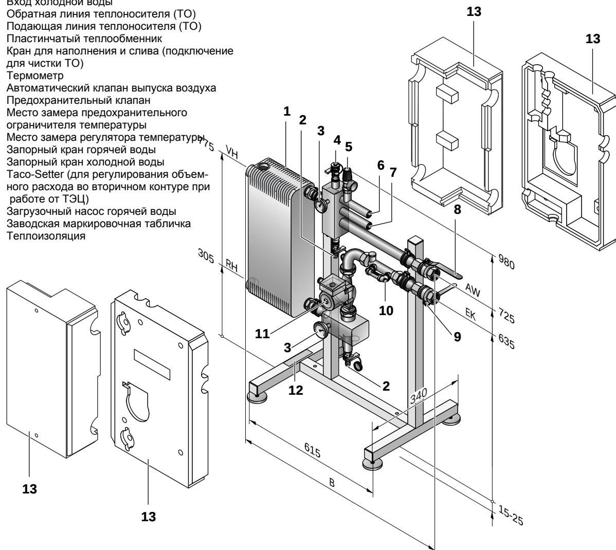
135/1 Размеры комплекта с промежуточным теплообменником Logalux LSP
